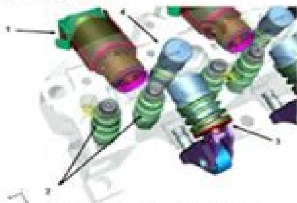
Fig. 5 Modulo Multiair (sezione per singolo cilindro)
