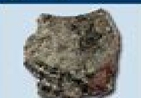
28. Sphalerite
