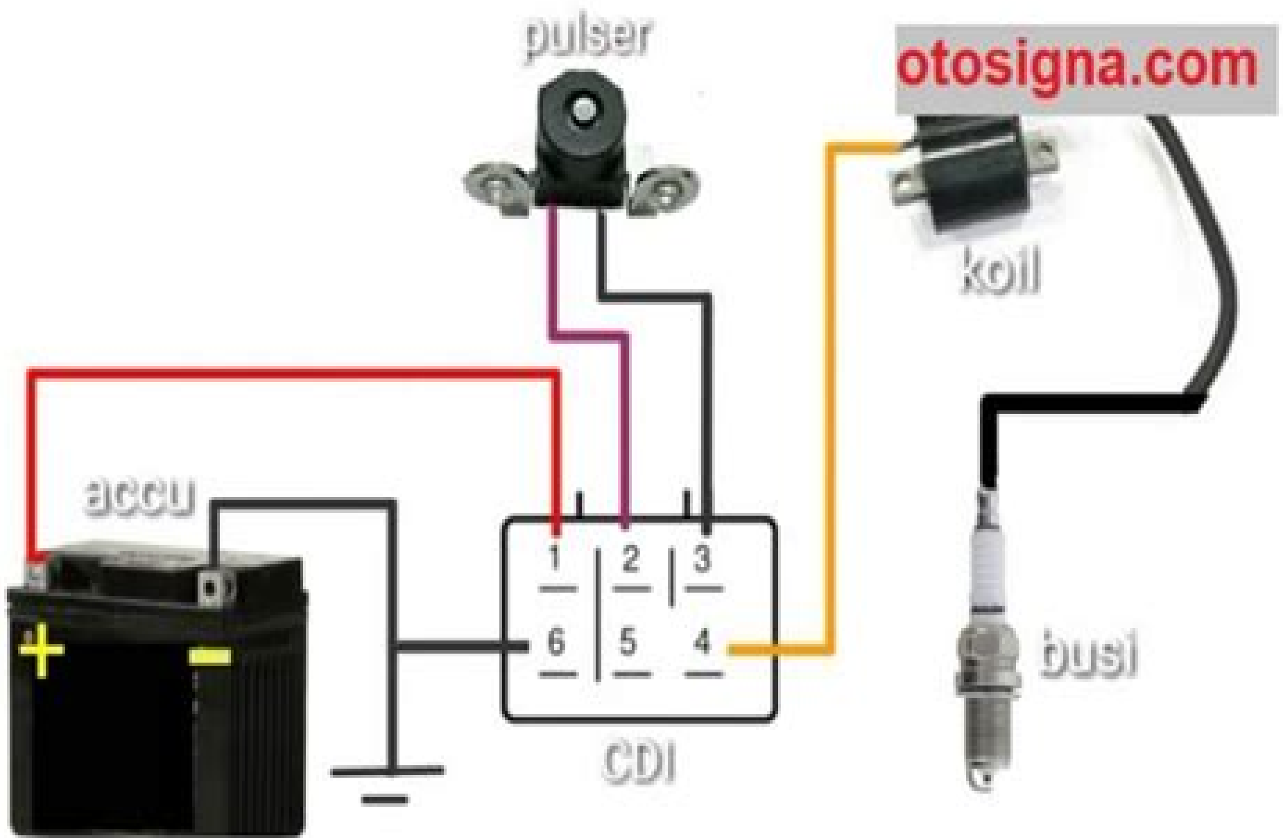
SISTEM PENGAPIAN SEPEDA MOTOR
