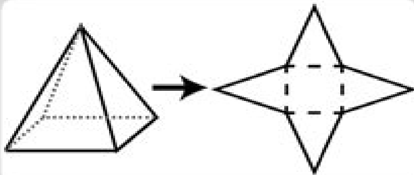
Right Pyramid
