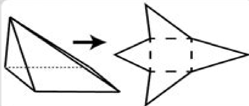
Oblique Pyramid
