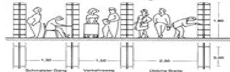
7 Mindestabstände
