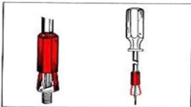
fig. 132 Spaninrichting voor route kappen.
