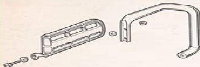
MONTAGGIO PARANNO MONTAGE DU PROTEGE-MAIN HAND GUARD ASSEMBLY ANSATZ DES HANDSCHUTZES MONTAGE DE PROTECTION
