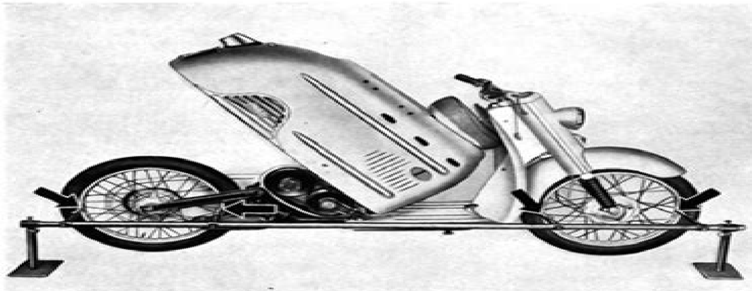
29 H: Sperrhebel beim Fluchten des Vorder- und Hinterrades
