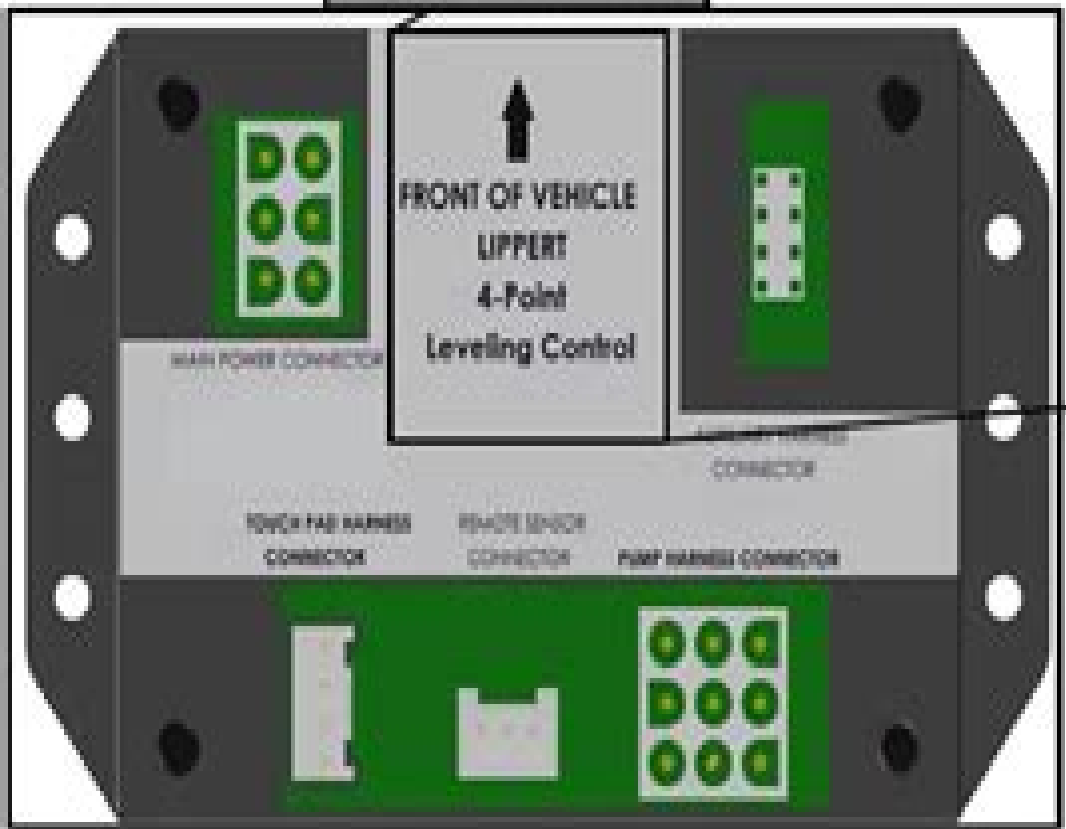
Fig. 2 - Controller
