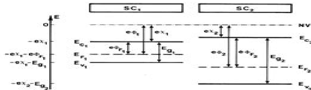
Figure 6-1 : Diagramme énergétique dans chacun des semiconducteurs
