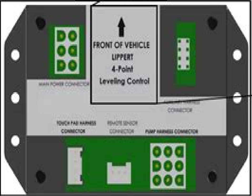
Fig. 2 - Controller
